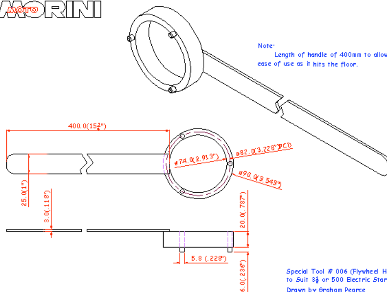
1. Special tool 006 - Attrezzo speciale 006
