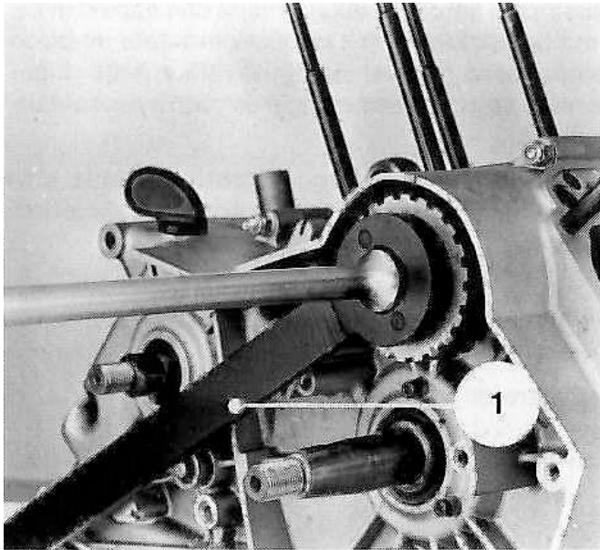
1. Special Tool 005 - Attrezzo speciale 005
