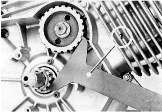
1. Special tool 009 - Attrezzo speciale 009
