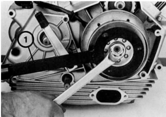
1. Special tool 006 - Attrezzo speciale 006
