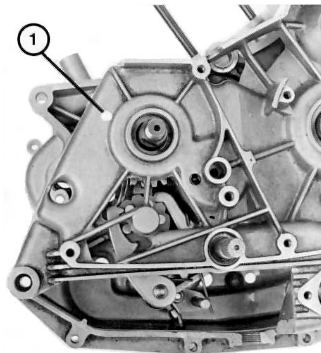
1. Special tool 008 - Attrezzo speciale 008
