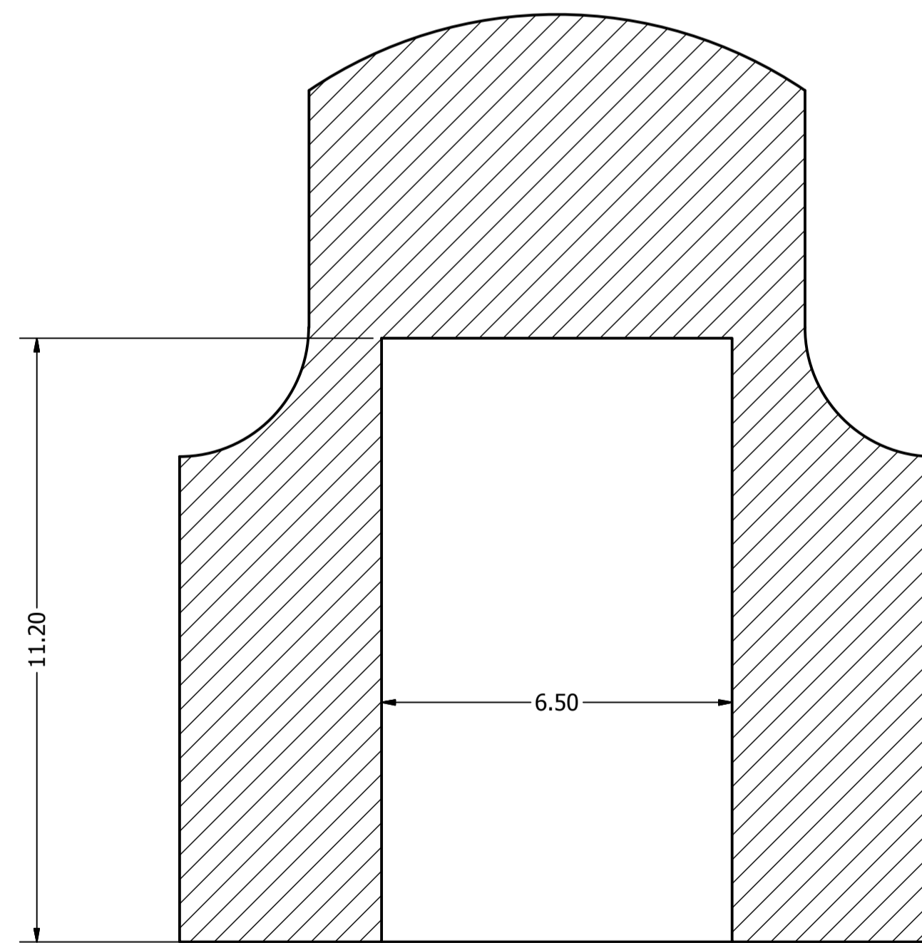
QUERSCHNITT A-A MASSSTAB 10 : 1
