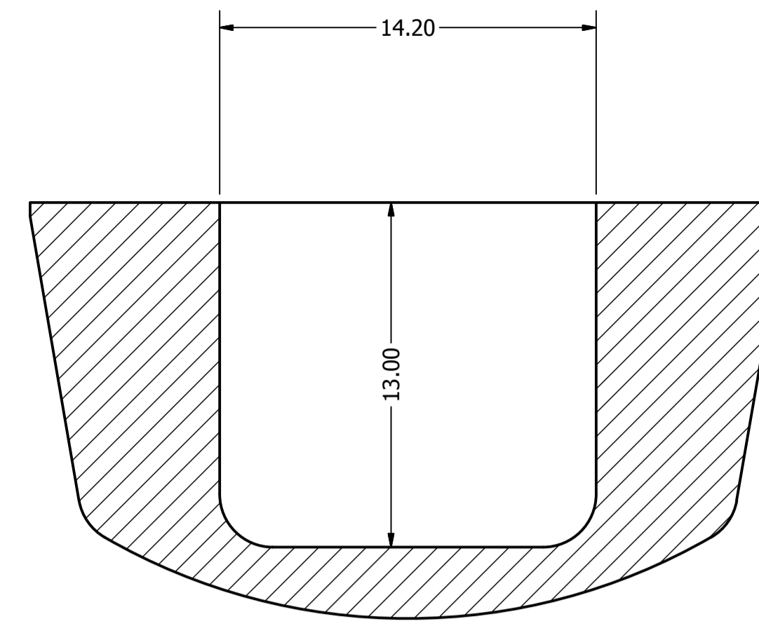
QUERSCHNITT A-A MASSSTAB 5 : 1
